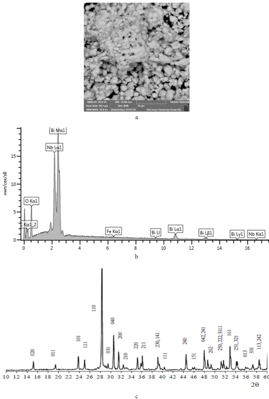
Рис. S1. Микрофотография поверхности (а), рентгеновский энергодисперсионный спектр (б) и дифрактограмма (с) образца \text{BiNb}_{0.97}\text{Fe}_{0.03}\text{O}_{4-6} .
