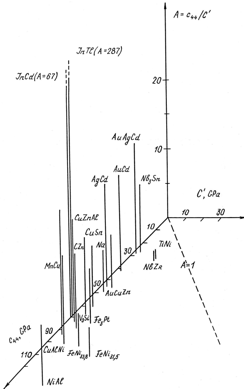
Рис. S1. Величина упругих постоянных c_{44} , C' и коэффициента упругой анизотропии A = c_{44}/C' кристаллов сплавов вблизи температур мартенситных превращений.
