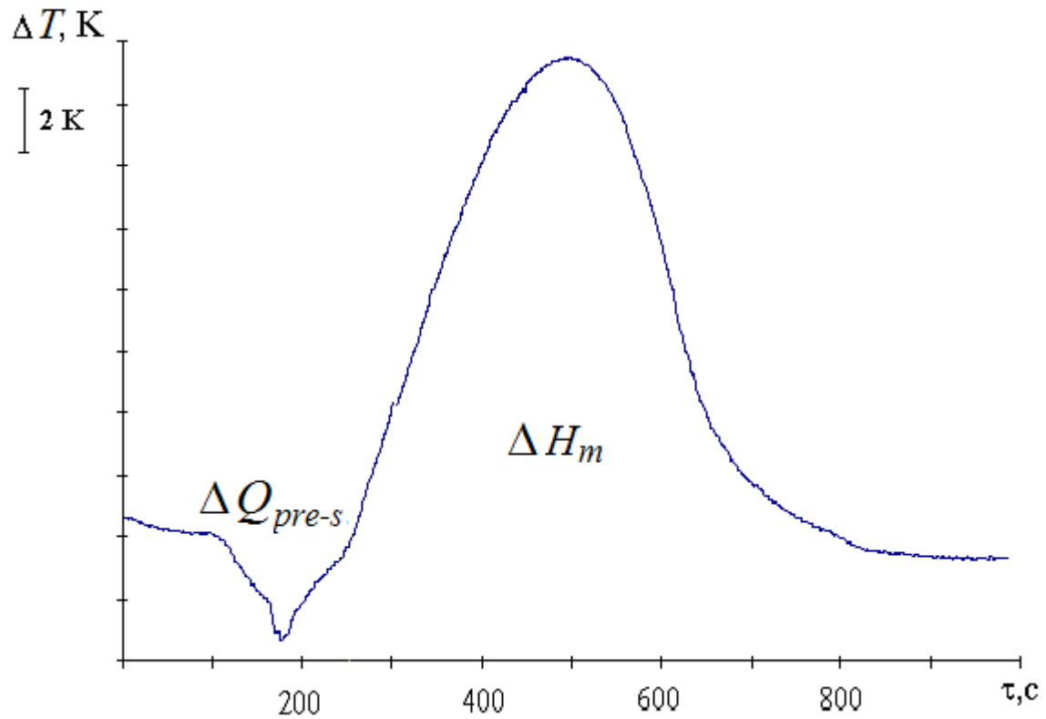
Рис. S2. Кривая ДТА кристаллизации KCl ( \nu = 5 K/min).
