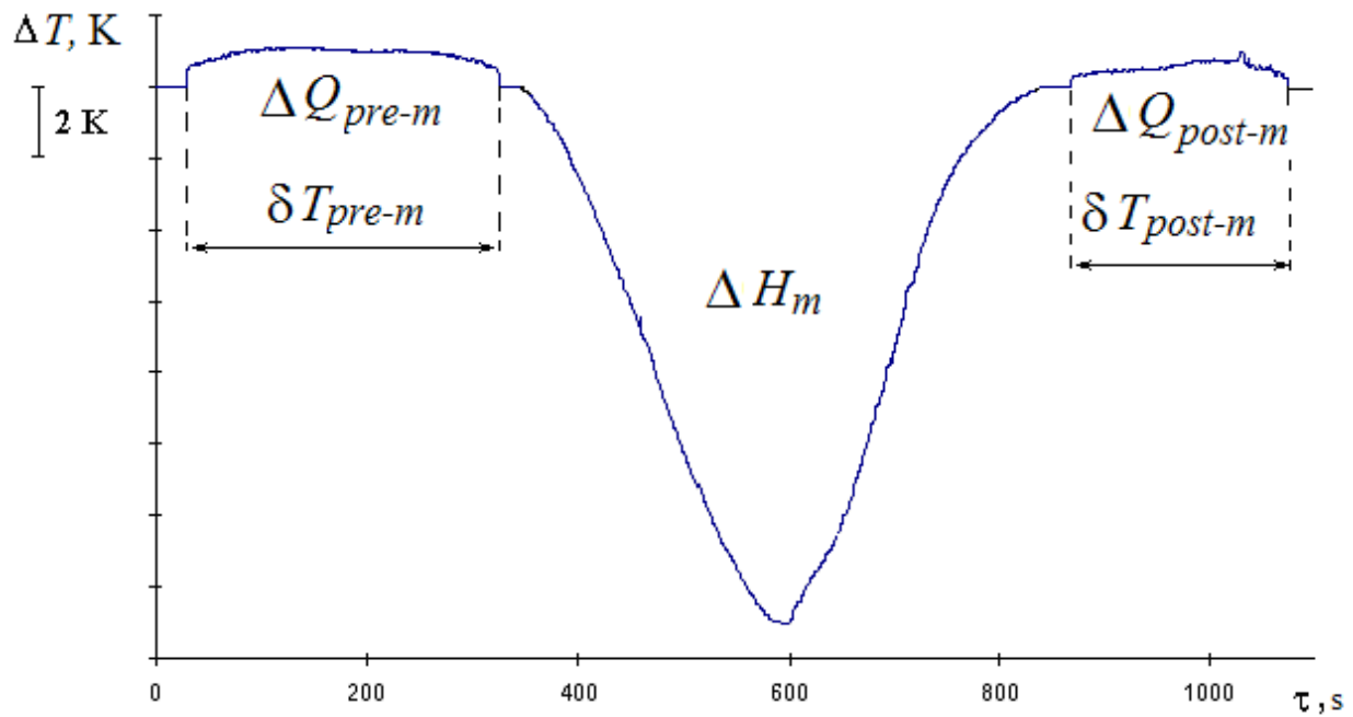
Рис. S1. Кривая ДТА плавления KCl ( \nu = 5 K/min).
