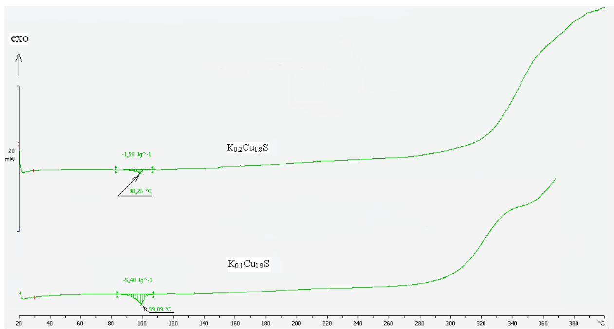
Рис. S2. Кривые дифференциальной сканирующей калориметрии для образцов K_{0.1}Cu_{1.9}S и K_{0.2}Cu_{1.8}S , полученные в атмосфере воздуха.
