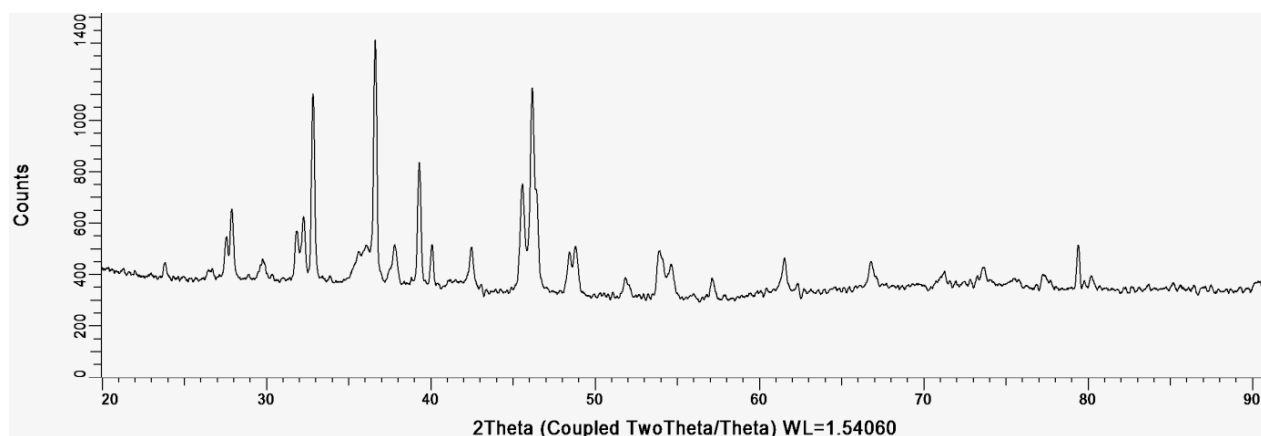
Рис. S1. Дифрактограмма образца K_{0.2}Cu_{1.8}S при комнатной температуре.
