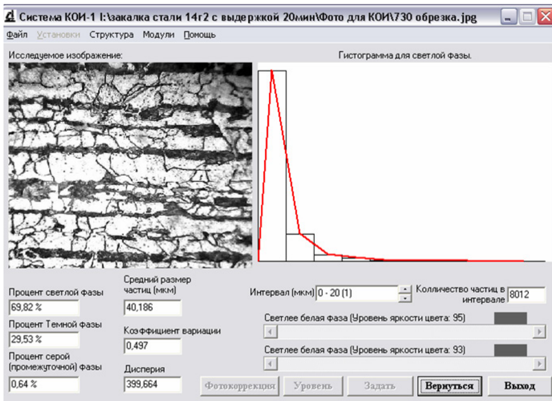
Fig. S1. Интерфейс программы КОИ-1 с примером результатов стереометрического анализа структуры ЕФМК стали 14Г2. Fig. S1. The interface of program KOI-1 with example of results of stereometric analysis of sample with NFMC structure.
