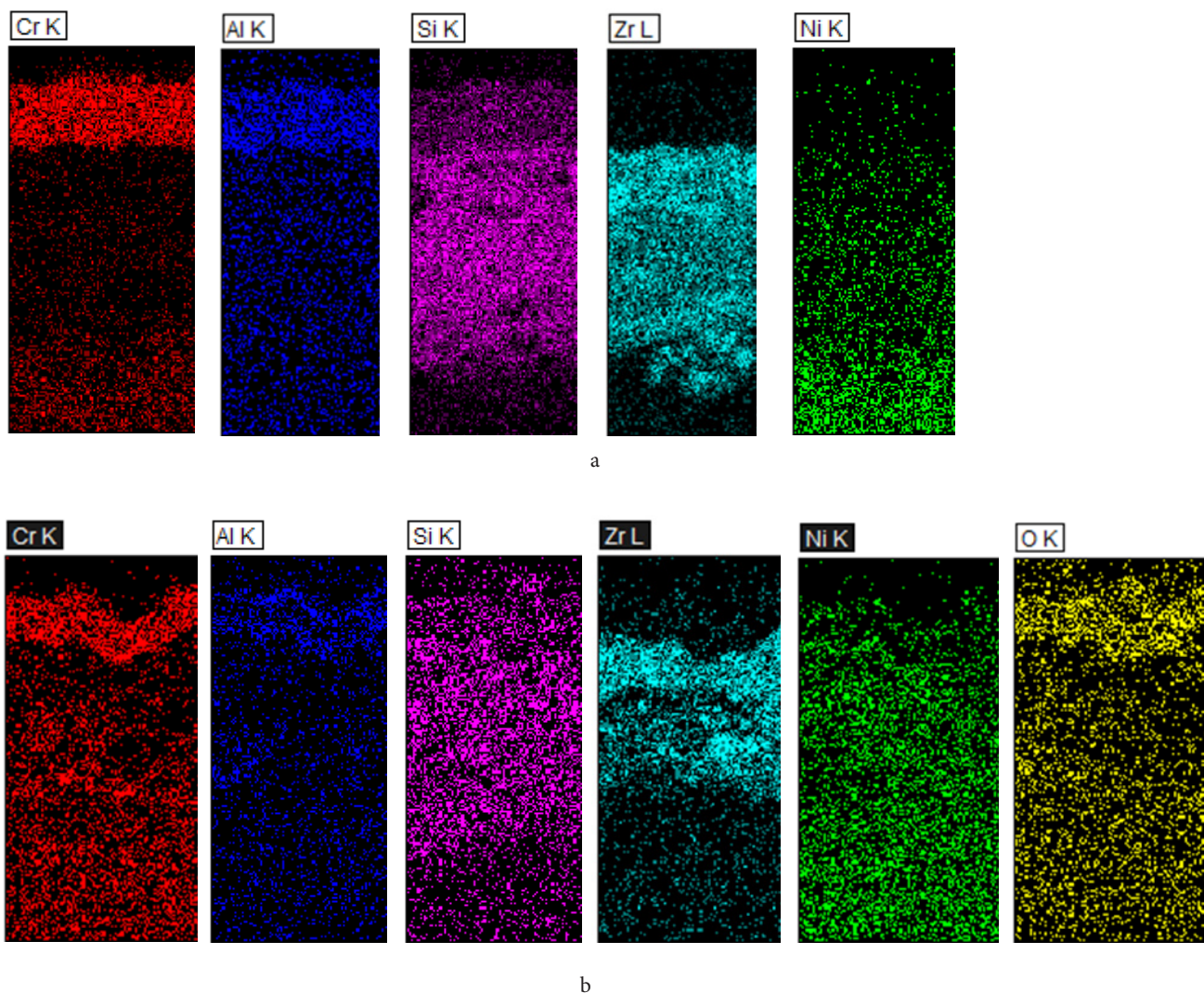
Рис. S3. (Color online) ЭДС-карты для двухслойного МН-ЭИЛ покрытия CrAlSiB/ZrSiB в исходном состоянии (а) и после отжига (б). Fig. S3. (Color online) EDS-maps for CrAlSiB/ZrSiB double-layer MS-ESA coating in the as-deposited state (a) and after annealing (b).
