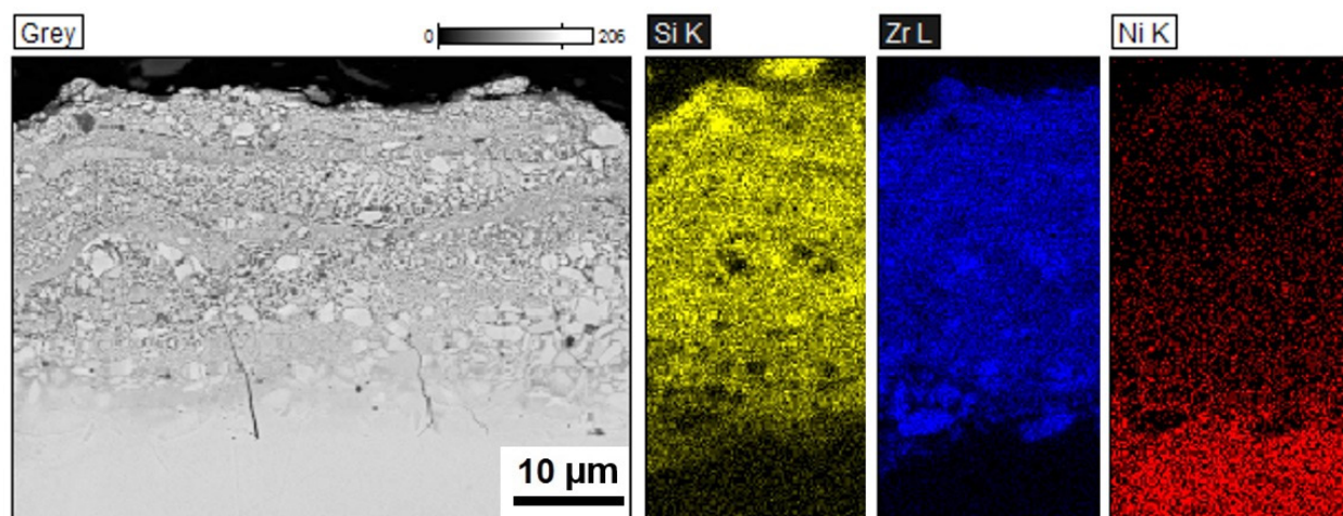
Рис. S1. (Color online) Данные СЭМ-ЭДС для однослойного ЭИЛ-покрытия ZrSiB.
