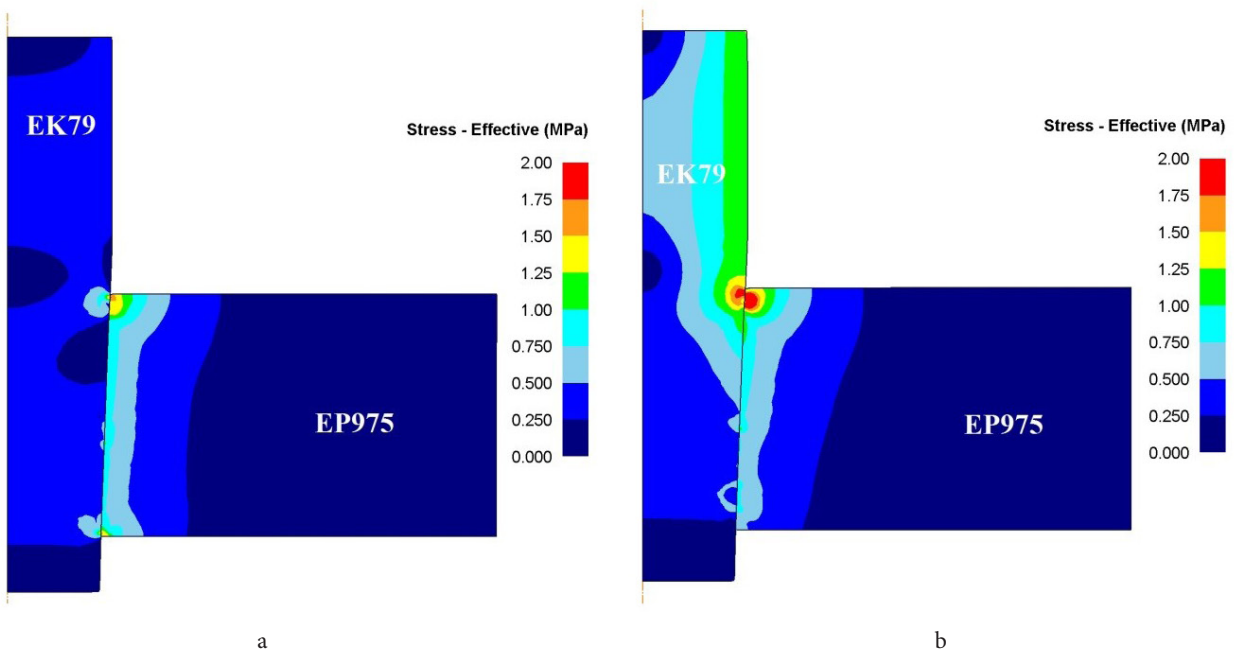
Рис. S2. (Color online) Распределение эффективных напряжений в вале (ЭК79) и диске (ЭП975) при СД по Схеме 1 (а) и Схеме 2 (б). Fig. S2. (Color online) The distribution of effective stress in the shaft (EK79) and disk (EP975) during pressure welding with a shear according to Scheme 1 (a) and Scheme 2 (b).
