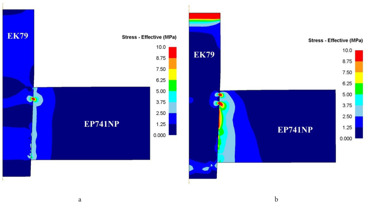
Рис. S1. (Color online) Распределение эффективных напряжений в вале (ЭК79) и диске (ЭП741НП) при СД по Схеме 1 (а) и Схеме 2 (б). Fig. S1. (Color online) The distribution of effective stress in the shaft (EK79) and disk (EP741NP) during pressure welding with a shear according to Scheme 1 (a) and Scheme 2 (b).
